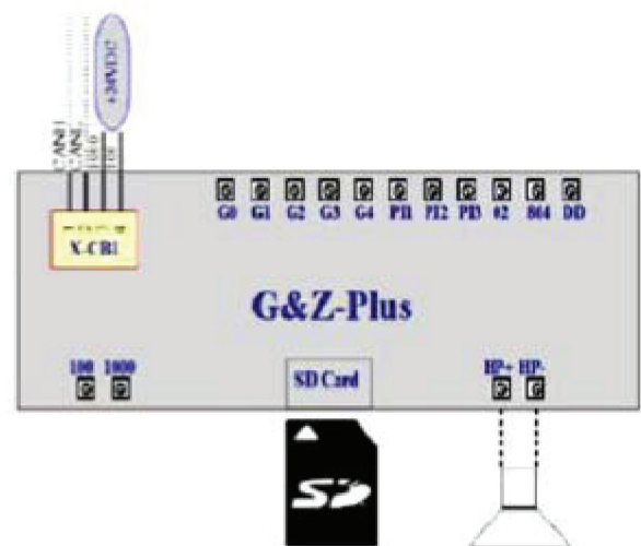
اتصال سری
