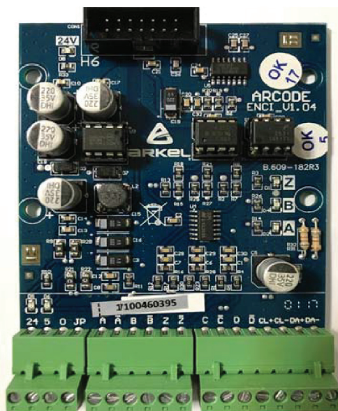
برد انکودر ENCI مربوط به موتورهای گیربکس
